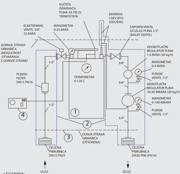
Schema kompletne isparivačke stanice SPI-12 (6-15 kg/h)
