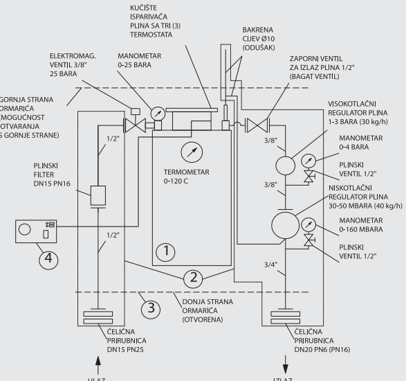
Schema kompletne isparivačke stanice SPI-24 (12-24 kg/h)
